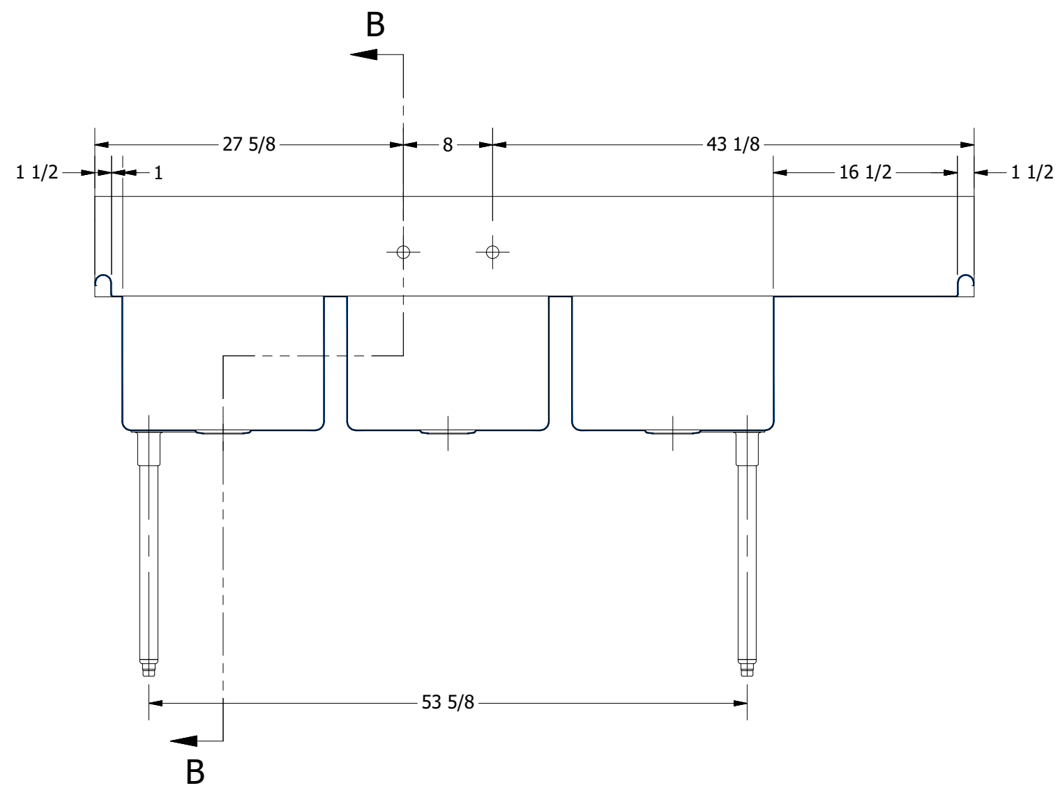
SECTION A-A SCALE 1:12
