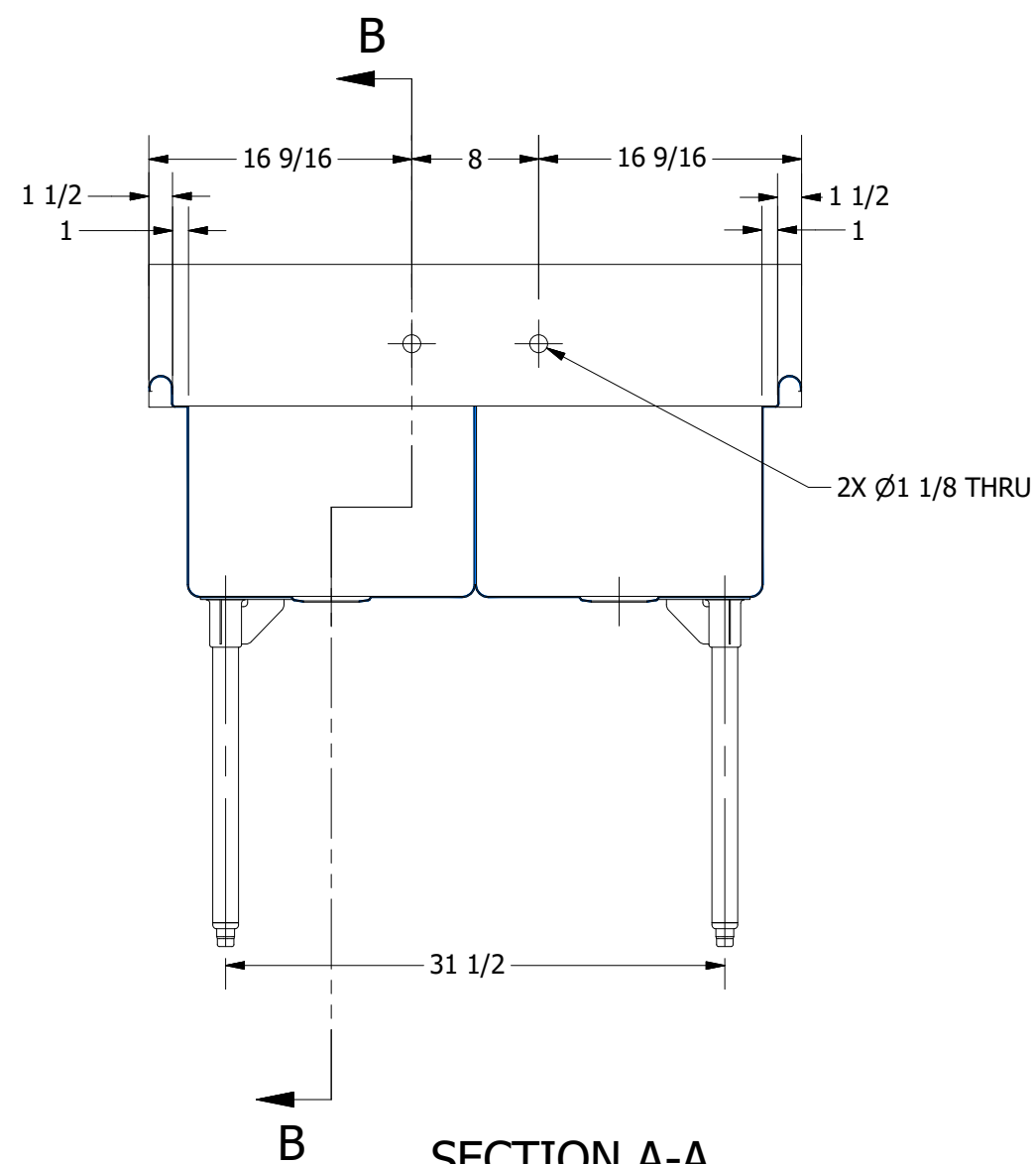
SECTION A-A SCALE 1:12
